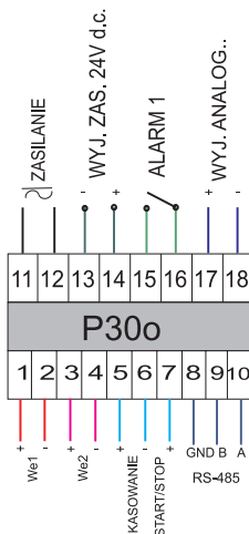
Rys.3. Schemat połączeń elektrycznych przetwornika w wykonaniach P30o-X12X01XX i P30o-X22X01XX
