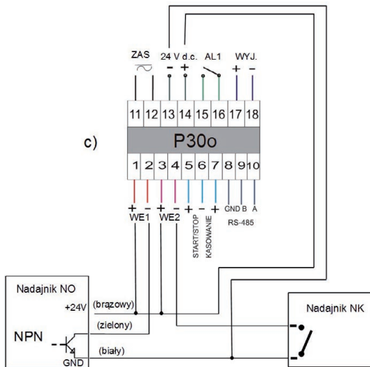
Rys.5. Schemat podłączenia wodomierza Powogaz z wyjściem nadajnika typu: a) kontaktron, b) optoelektroniczne, c) z oboma wyjściami.
