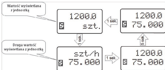
Rys 24A. Algorytm wyświetlania dwóch wartości z jednostkami.
